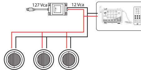
DIAGRAMA ILUSTRATIVO DE CONEXIÓN
